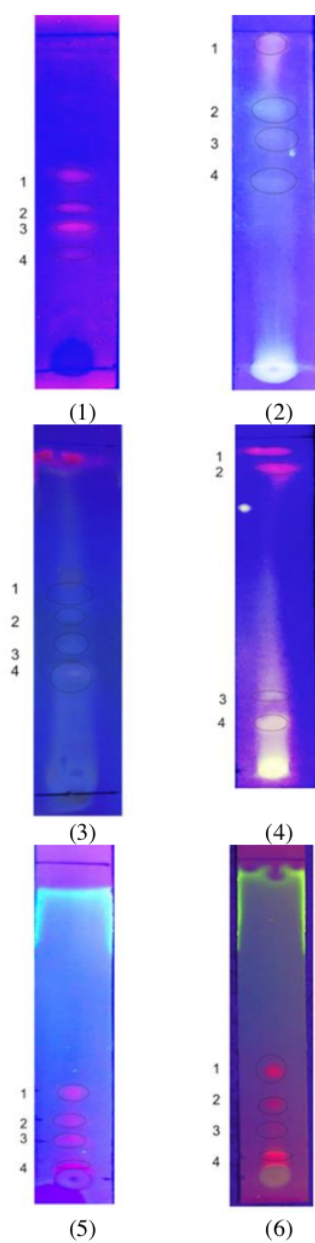
Gambar 2. Profil KLT pada pengamatan di bawah sinar UV 366 nm dari ekstrak etanol daun gedhi untuk berbagai metabolit sekunder (1) alkaloid (2) polifenol (3) flavonoid (4) tanin (5) saponin (6) steroid
