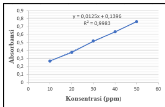
Gambar 3. Kurva Kalibrasi Asam Galat
