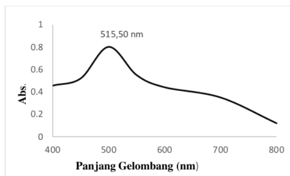
Gambar 4. Panjang Gelombang DPPH
