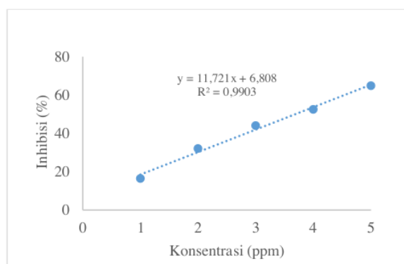
Gambar 5. Kurva Kalibrasi Vitamin C
